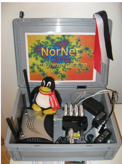
A NorNet Edge Node
